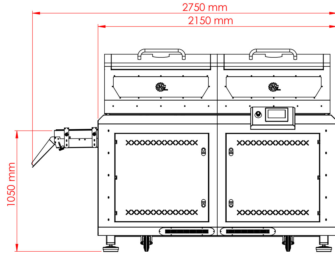
KESIT A-A
